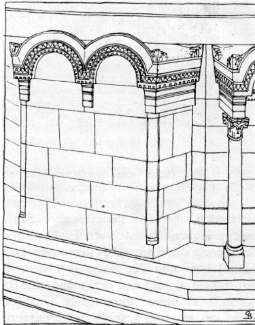
Bild 20. Die Ostseite des oberen Zehneckes. Ursprünglicher Zustand.
