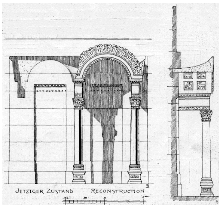
Bild 15. Die acht gleichen Wände des Obergeschosses.
