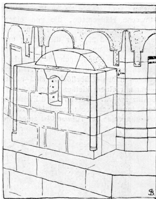
Bild 19. Die Ostseite des oberen Zehnecks. Jetziger Zustand.
