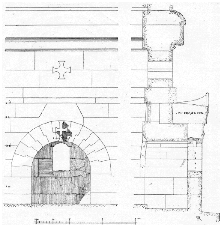
Bild 25. Die Nische in der Ostwand des Obergeschosses, Innenansicht und Schnitt.
