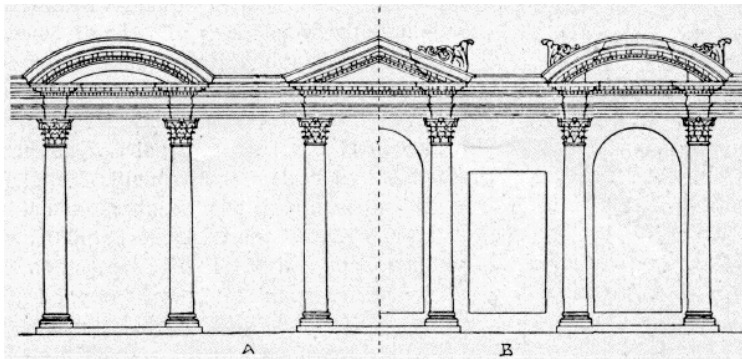
Bild 11. Schema einer Ädiculenreihe, in zwei Variationen.
