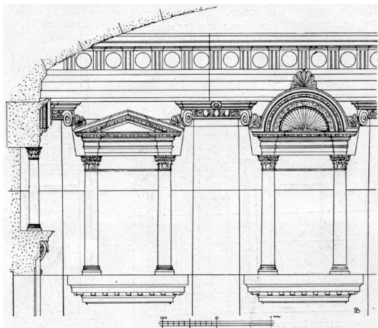
Bild 16. Aedicula und Conche mit besonders eingesetzten Steinen für die Verdachungen, aus den Substruktionen des grossen Tempels in Baalbeck.
