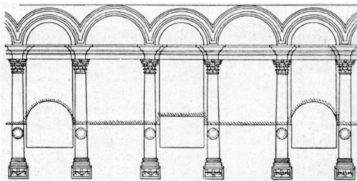
Bild 12. Conchenreihe der Porta aurea des Diokletianpalastes in Spalato.
