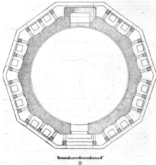
Bild 24. Grundriss des Obergeschosses, rekonstruiert von Bruno Schulz.
