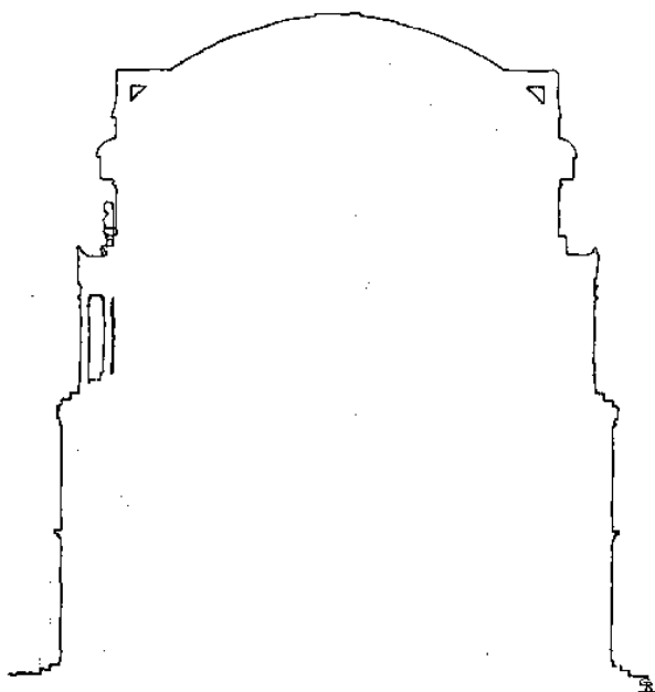
Bild 21. Das Theoderich-Grabmal von Süden gesehen. Ursprüngliche symmetrische Umrisslinie.
