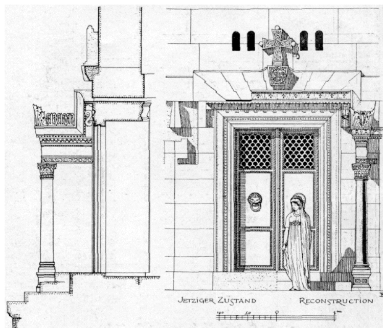
Bild 22. Die Türwand des Obergeschosses.
